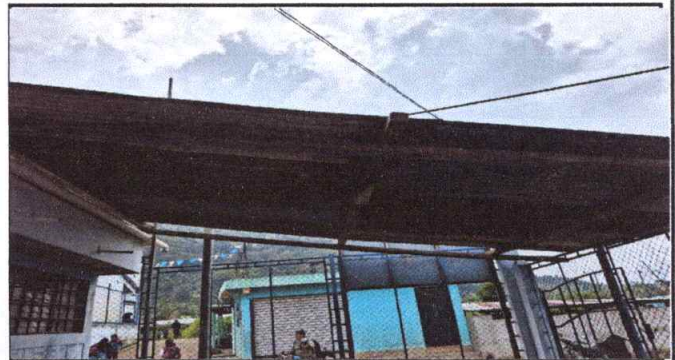
Foto 2: MODULO II. PATIO: Sustitución de estructura de soporte de madera y lámina por soprte de metal y lamina troquelada aluzinc calibre 26. 6 tubos de 4x4 chapa 16, 4 tubos rectangulares 2x6 chapa 16, 12 tubos 2x2
